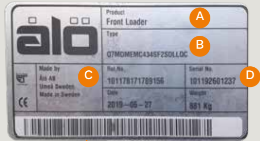
Plaque d'identification chargeur
