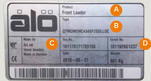
Maskinskylt för redskap
