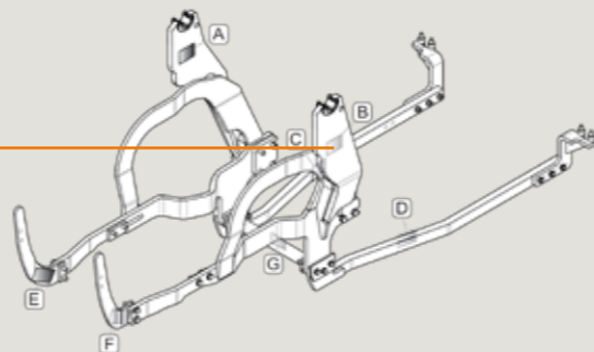
Dekaler med artikelnummer på fundamentets komponenter
