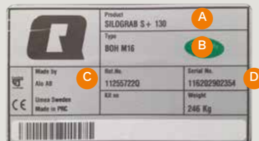
Työlaitteen konekilpi
