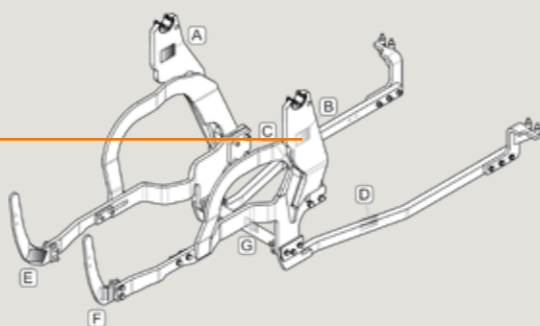
Siirtokuvat tuotekoodin kanssa apurungon komponenteissa
